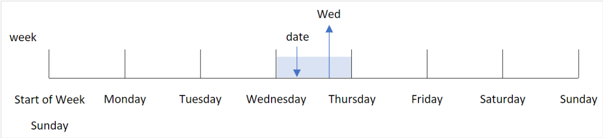
返回日期所在日期名称的 weekday() 函数图表
