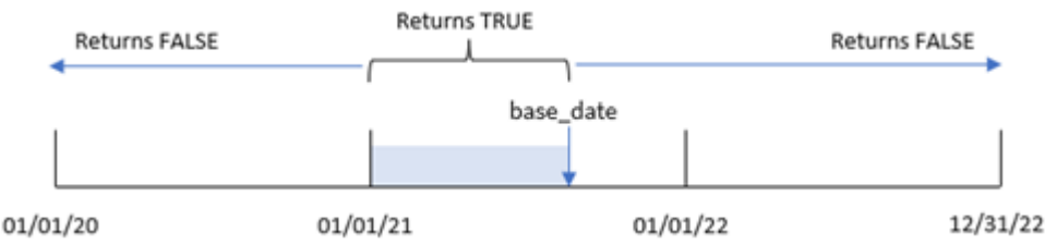
inyeartodate 函数图表
