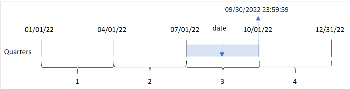
quarterend() 函数的图表
