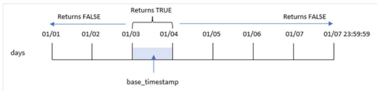
inday 函数的图表
