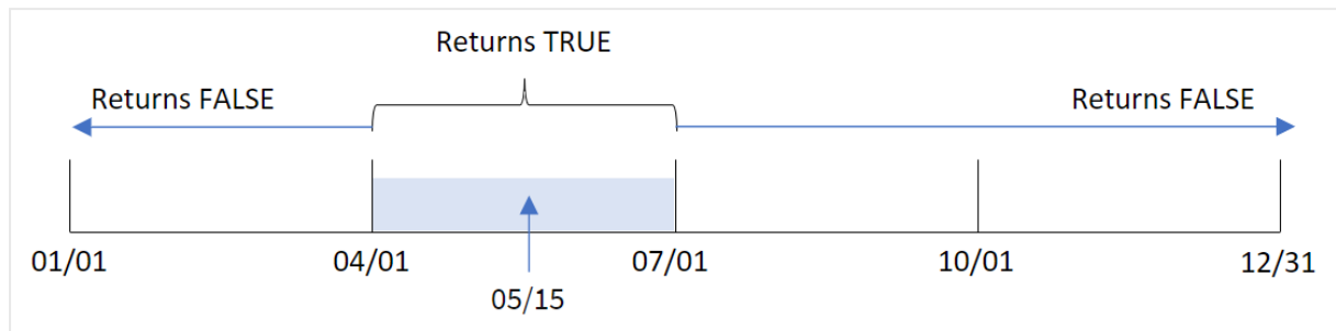
带季度段的 inmonths() 函数的图表
