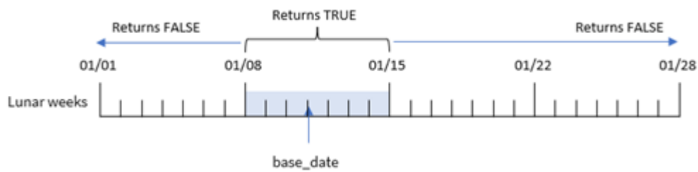
inlunarweek() 函数的图表
