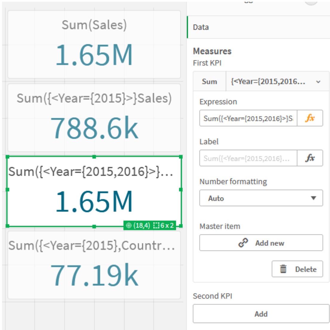
使用集合修饰符的 KPI
