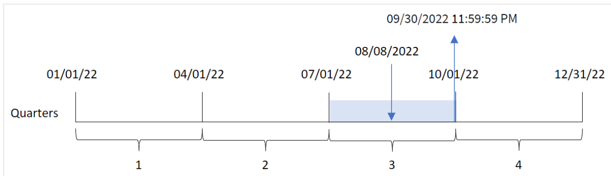
Диаграмма функции quarterend() , определяющей конец квартала для транзакции 8203
