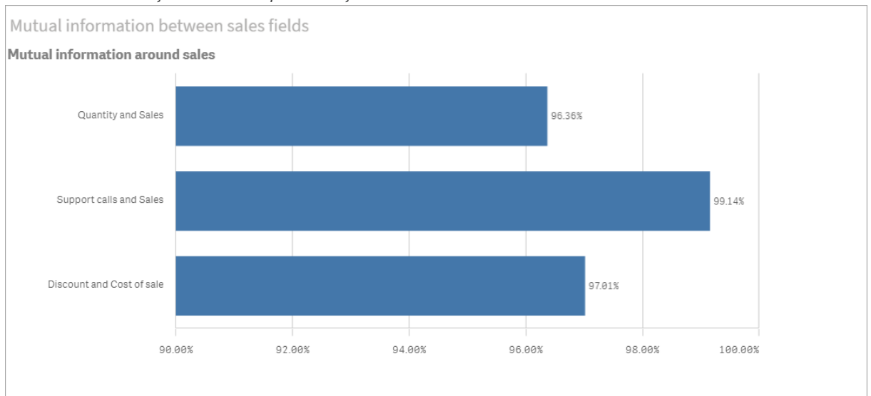
Gráfico de informações mútuas após a edição
