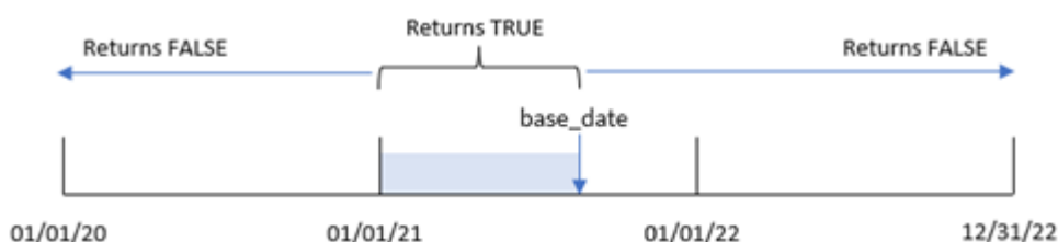
Diagram funkcji inyeartodate
