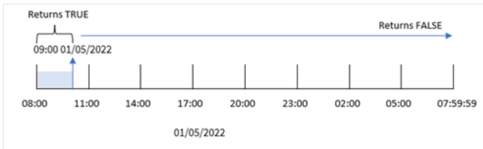
예 3 오전 8시부터 오전 9시까지 트랜잭션이 있는 indaytotime 함수 다이어그램,
