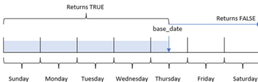
Diagramme de la fonction inweektodate
