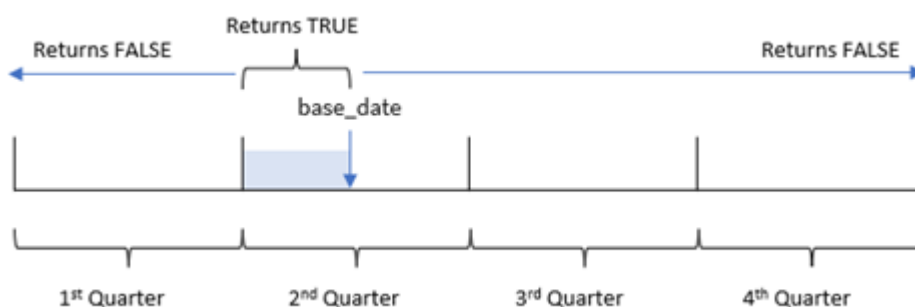
Diagramme de la fonction inquartertodate
