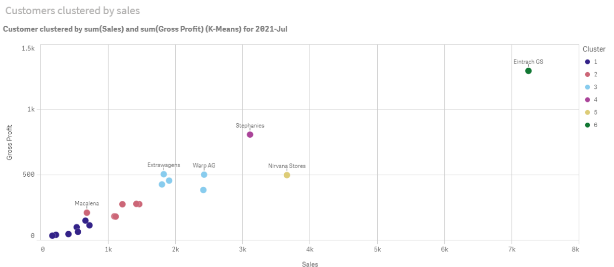
Graphique Nuage de points KMeans après éditions
