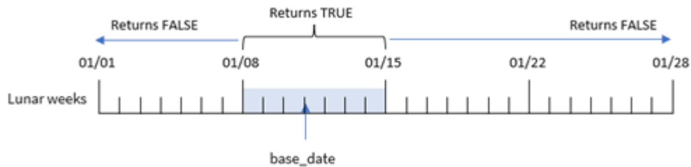
Diagrama de la función inlunarweek()
