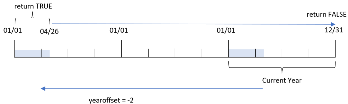
Diagramm der Funktion yeartodate() , Beispiel „yearoffset“
