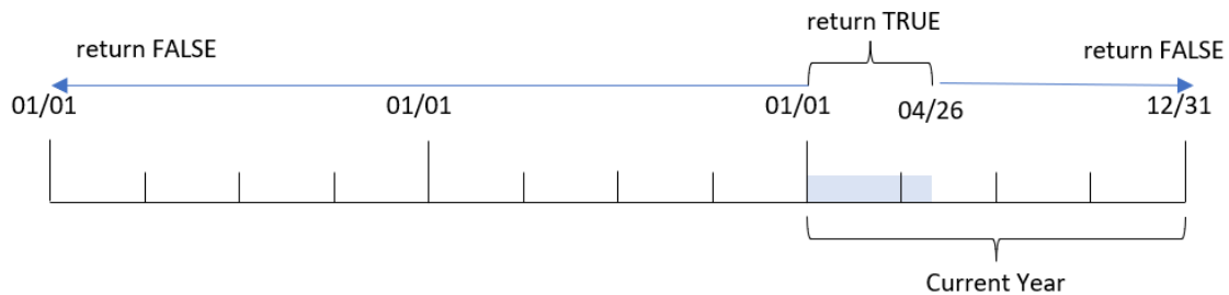
Diagramm der Funktion yeartodate() , Diagrammobjektbeispiel
