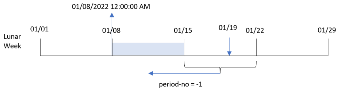
Diagramm der Funktion lunarweekstart() , Beispiel „period_no“
