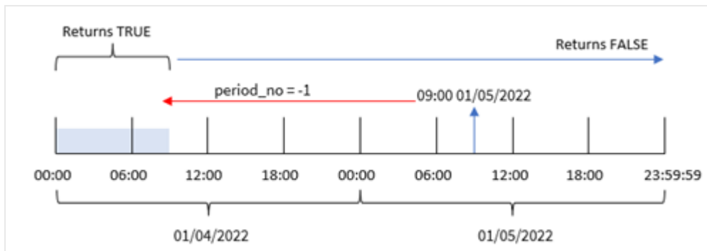
Beispiel 2: Diagramm der Funktion indaytotime mit Transaktionen ab dem 4. Januar
