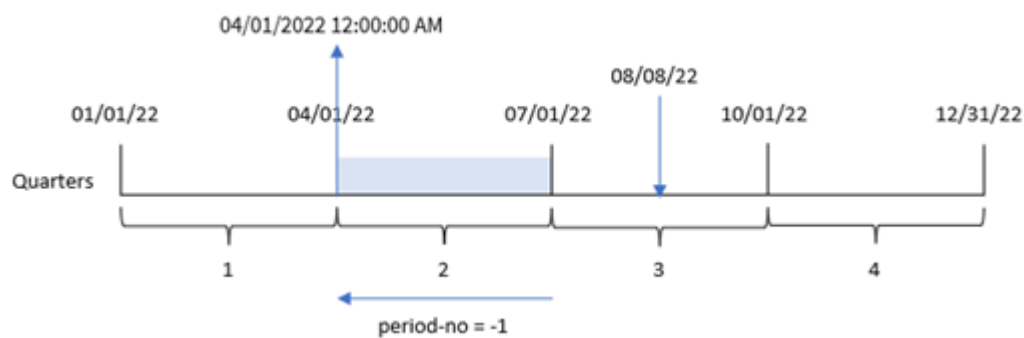
Diagramm der Funktion quarterstart() , Beispiel „period_no“
