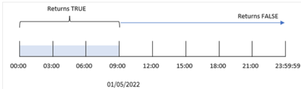
Beispiel 1: Diagramm der Funktion indaytotime mit 9:00-Uhr-Limit.
